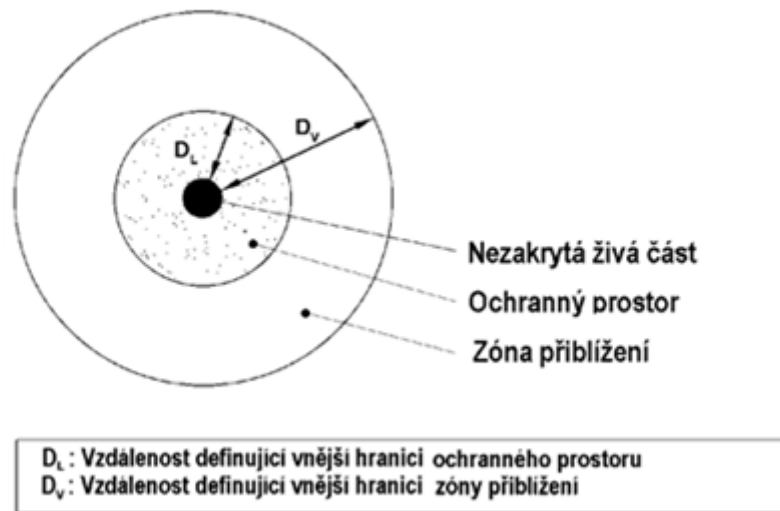
Obrázek 1 - Vzdušné vzdálenosti a zóny pro pracovní postupy
